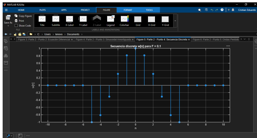
Figura 13: Secuencia discreta w[n] para F = 0,1 .
