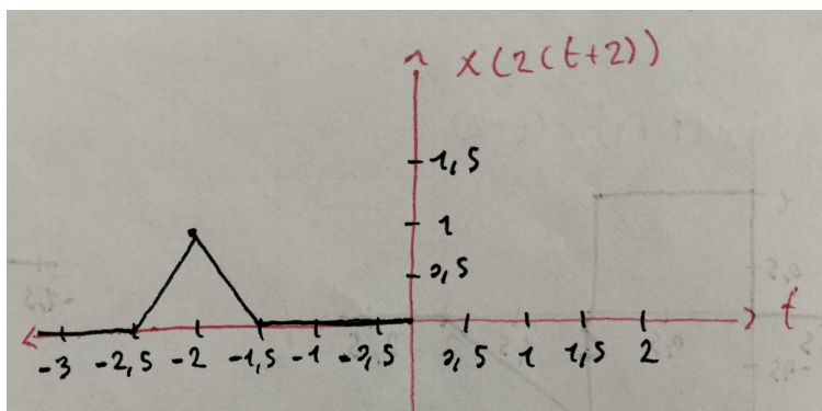
Figura 2: Señal x(2(t+2))
