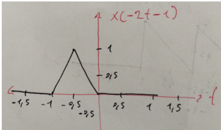
Figura 1: Señal x(-2t - 1)
